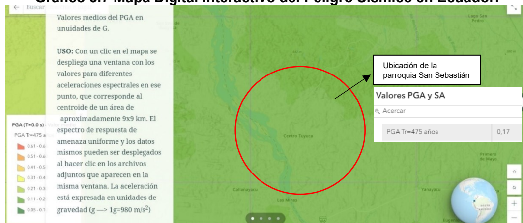
Gráfico 3.7 Mapa Digital Interactivo del Peligro Sísmico en Ecuador.
