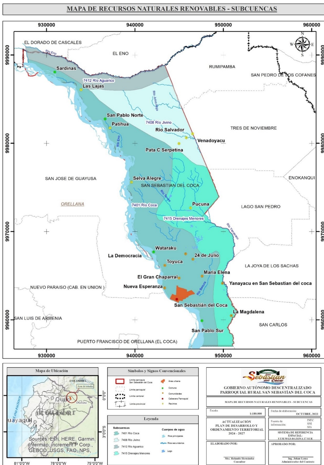
Mapa 3.4 Mapa de recursos naturales renovables – subcuencas
