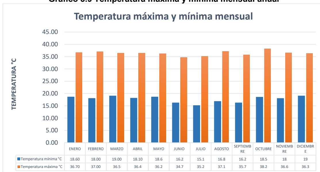
Gráfico 3.9 Temperatura máxima y mínima mensual anual
