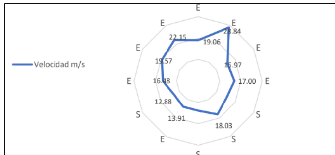
Gráfico 3.16 Velocidad media m/s
