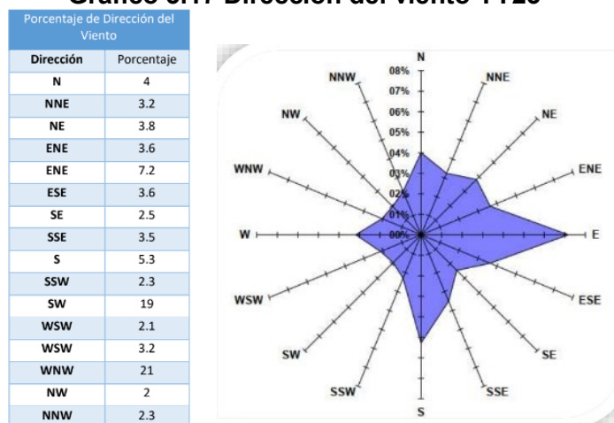
Gráfico 3.17 Dirección del viento YY23
