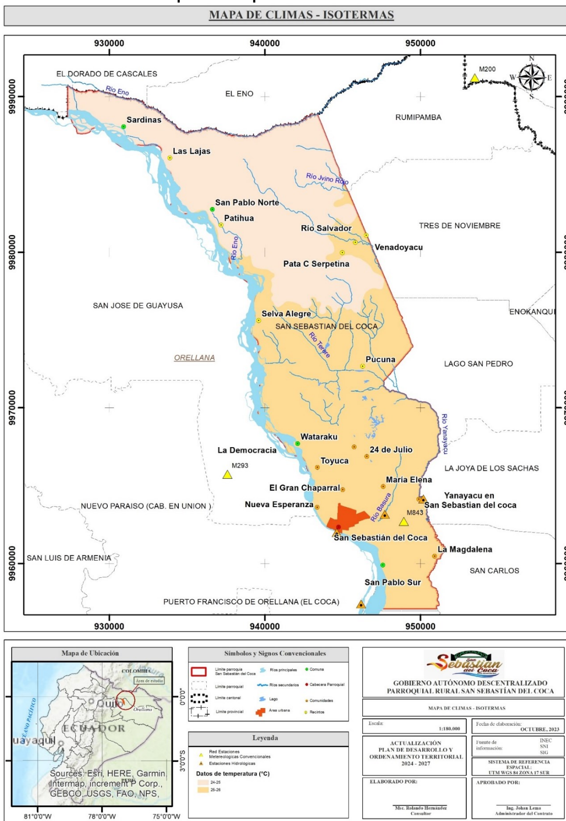
Mapa 3.16 Mapa de climas– Isotermas
