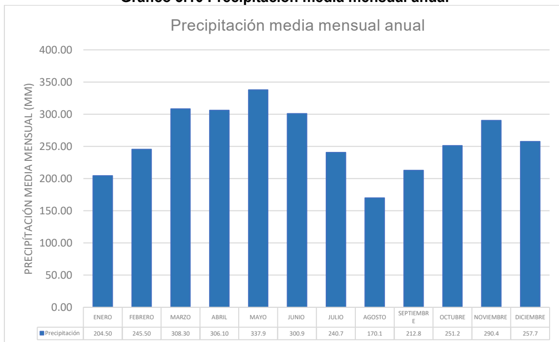
Gráfico 3.10 Precipitación media mensual anual
